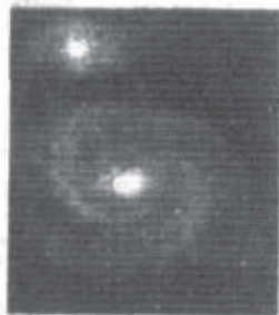
Una galaxia doble
